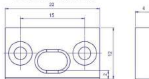
Schließblech
