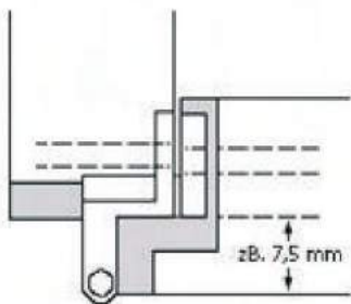
Superfalz
