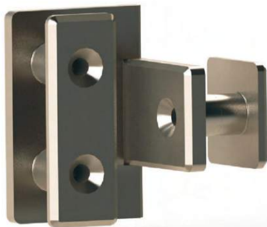
Innenansicht
